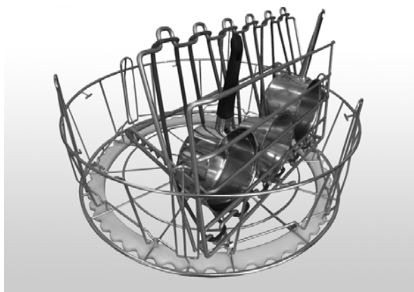
Obrázek 11: Víceúčelový držák
